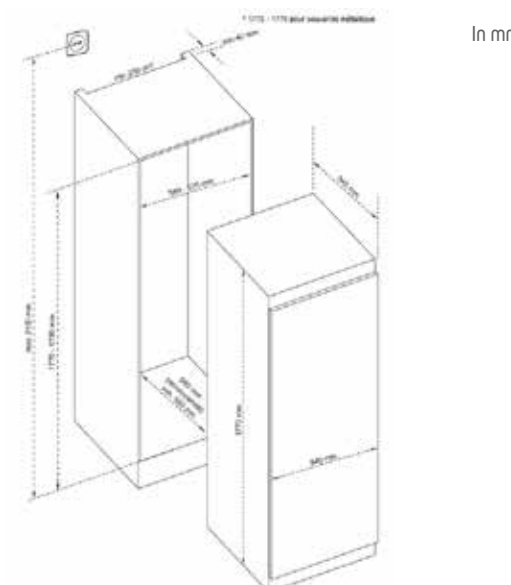
BIL1770EB scheme
