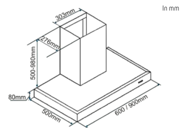
AD1516X 60cm scheme
