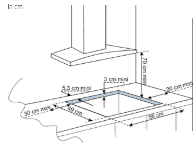
BPG6414B & BPG6413W/B Glass Hobs scheme
