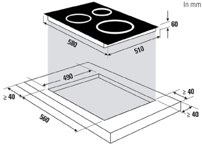
BPI6414BM 60cm scheme
