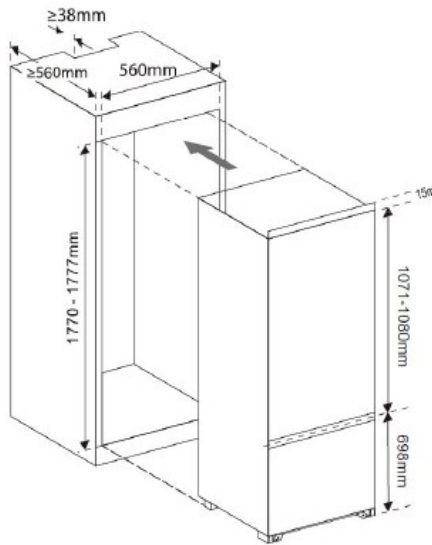
BIC1724ES scheme
