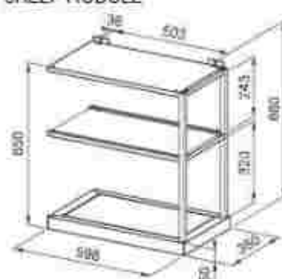
SHELF MODULE
