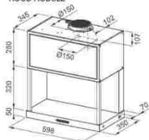
HOOD MODULE
