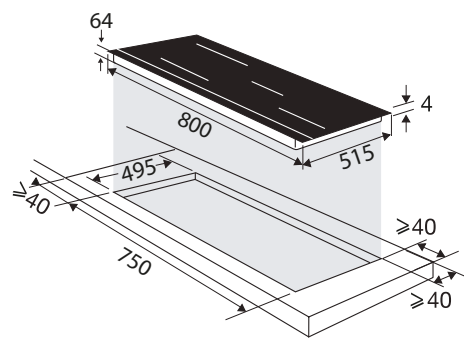
Encastrement sur plan table 800
