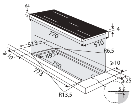
Encastrement à fleur table 800
